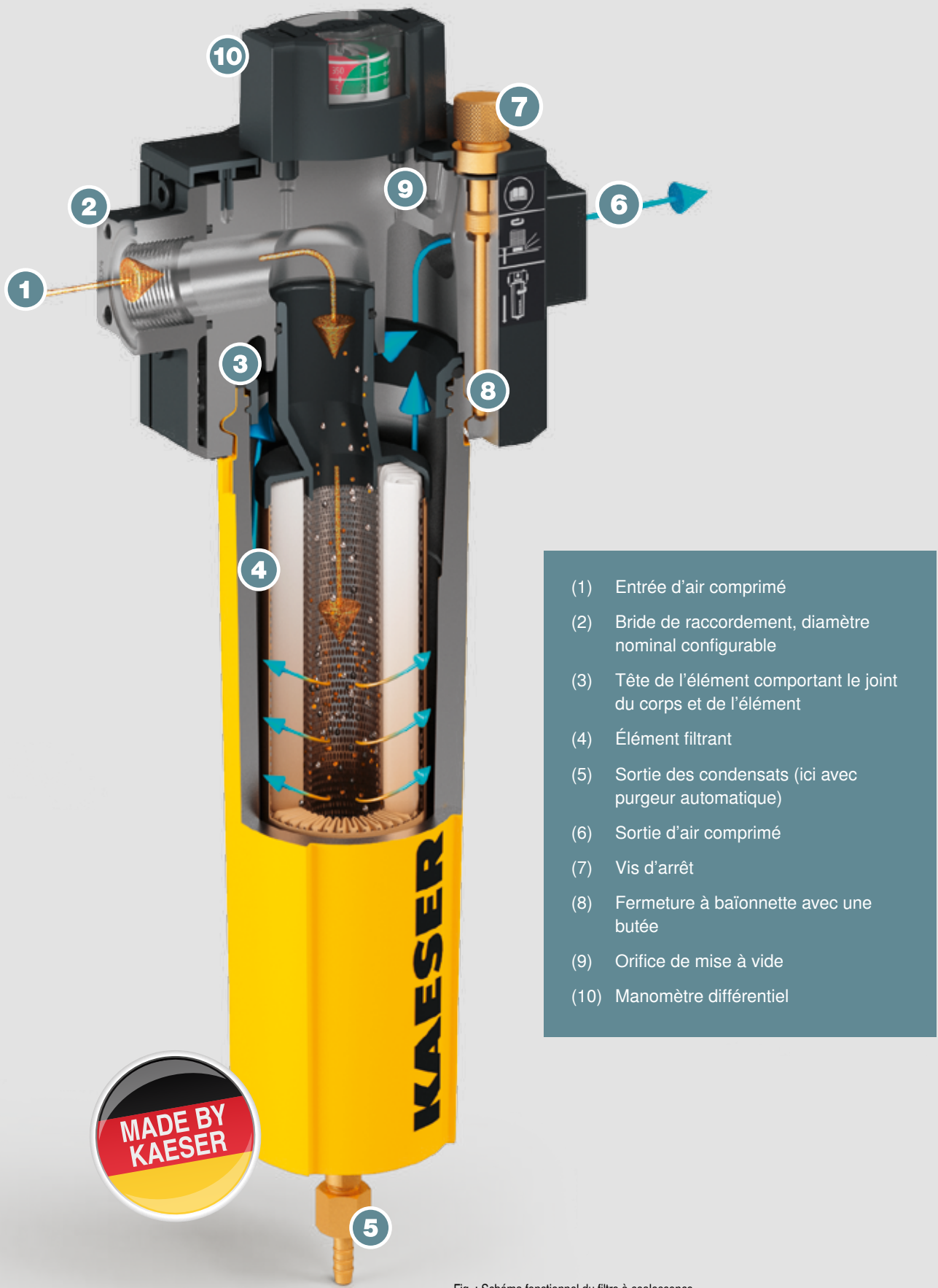
Fig. : Schéma fonctionnel du filtre à coalescence
