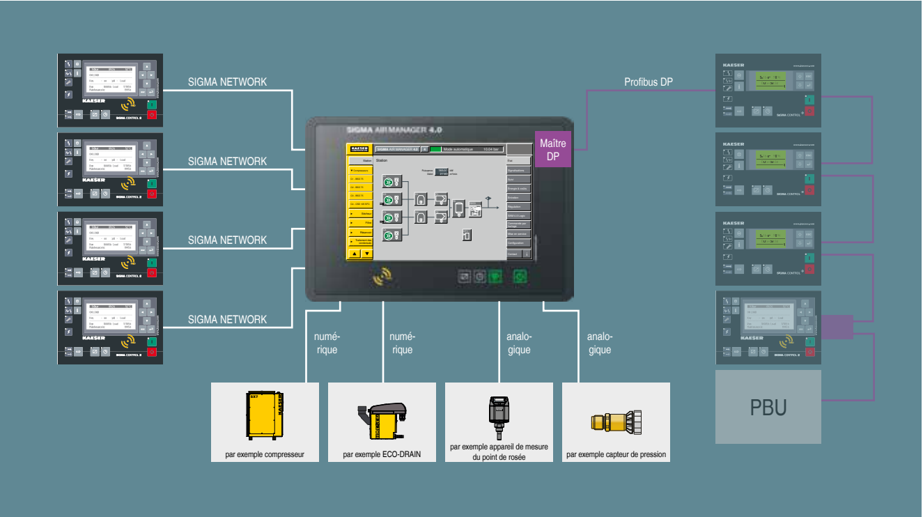
Station d'air comprimé gérée par le SIGMA AIR MANAGER 4.0 – Raccordements possibles
