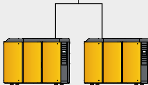
Connexion des compresseurs équipés du SIGMA CONTROL 2
